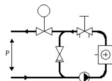
B. Typowy układ z lokalną pompą cyrkulacyjną
