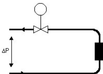
A. Typowy układ bez lokalnej pompy cyrkulacyjnej
